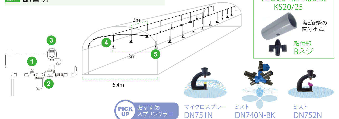
【しいたけ菌床栽培 設置例】
