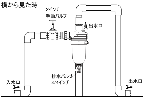
【AKY388】配管例
