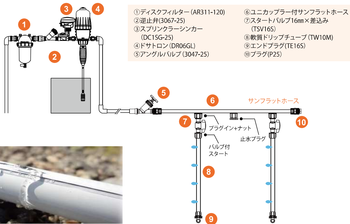
図23 軟質ドリップチューブによるドリップファーターゲーション 配管例
