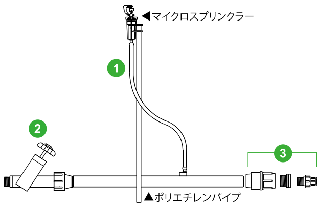
図18 ポリ式配管例
