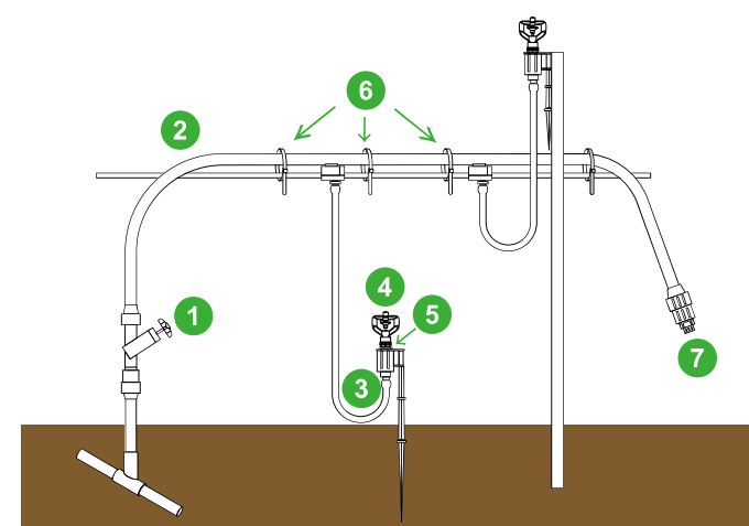
図07 棚配管例
