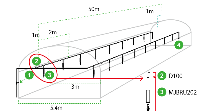
図04 ポリ式配管例
