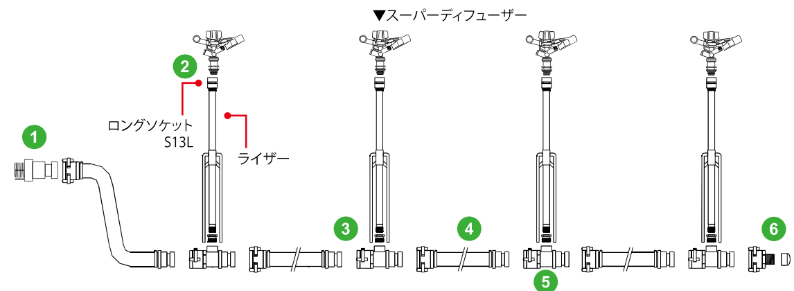
図20 セット内容配管例
