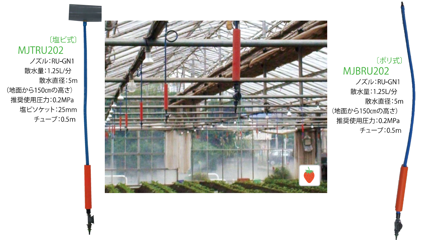
図03 塩ビ式配管例
