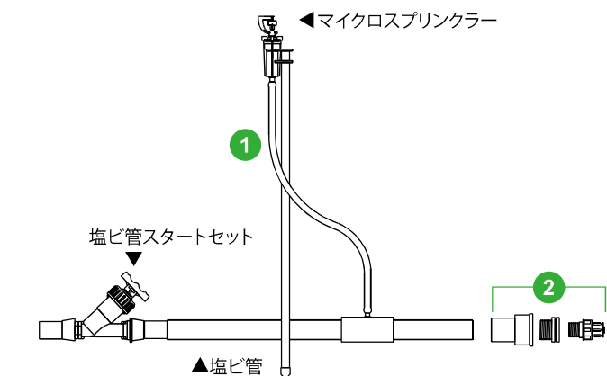
図17 塩ビ式配管例
