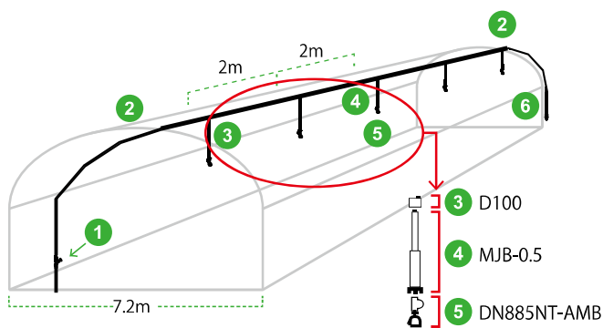
図02 ポリ式配管例
