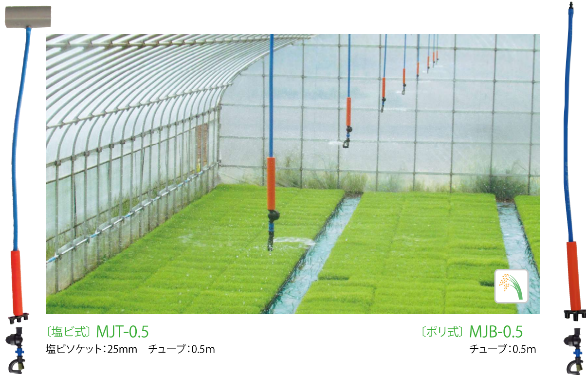
図01 塩ビ式配管例
