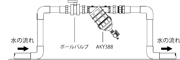
【AKY388】配管例
