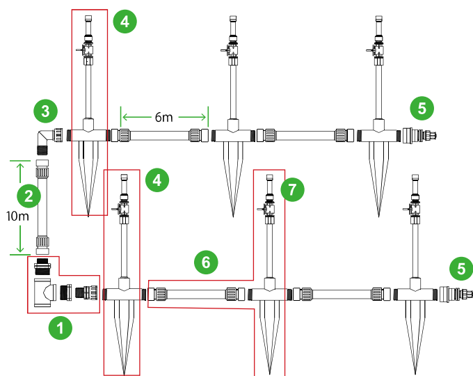
図14 配管例
