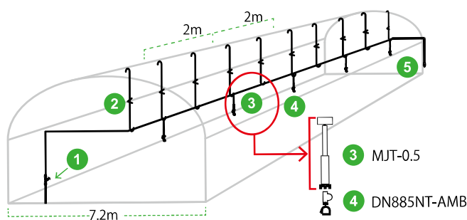
図01 塩ビ式配管例
