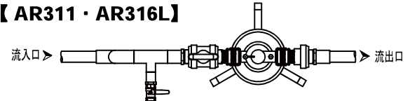
塩ビ配管 標準取付図
