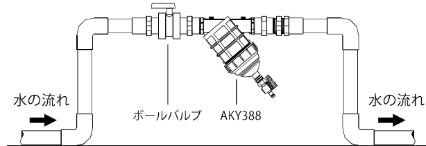
【AKY388】配管例
