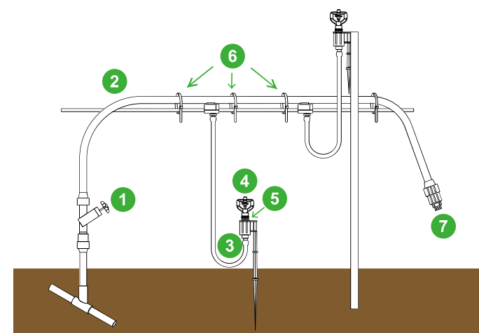
図07 棚配管例
