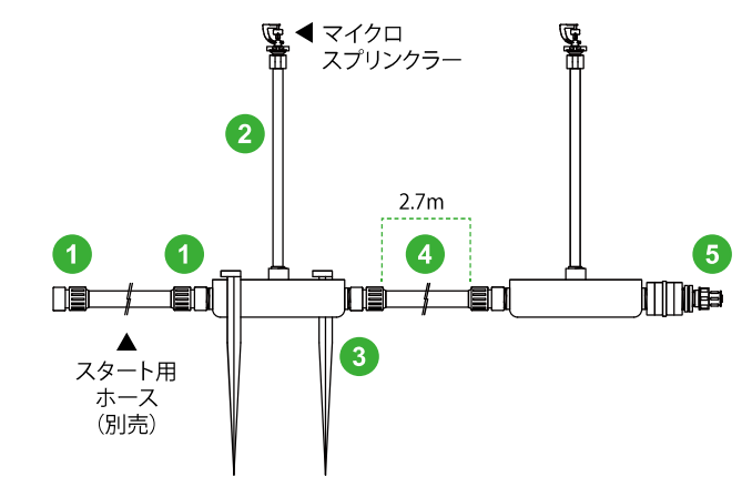
図16 プレート式配管例
