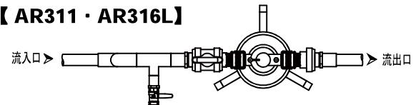
塩ビ配管 標準取付図
