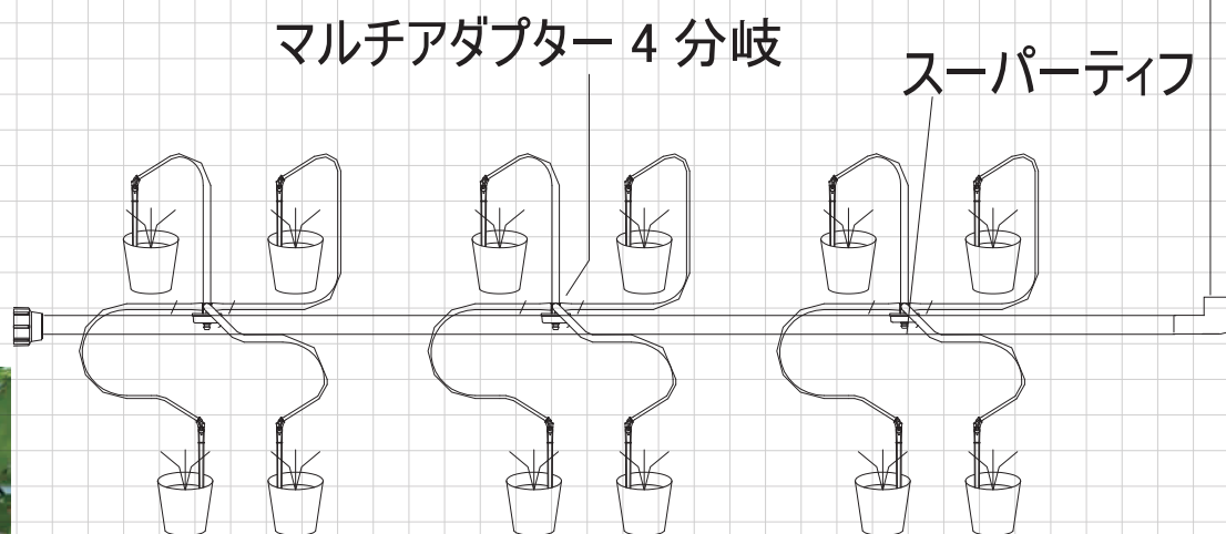
◀ マルチアダプター 4 分岐
